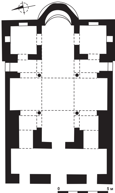
6. Храм Н в Сиде. План
