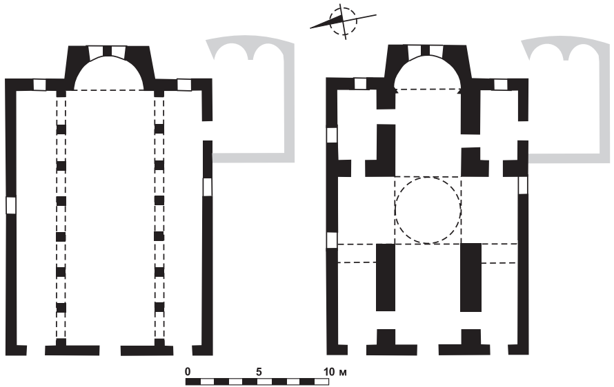
17. Храм в Кидне (Пидне). План
