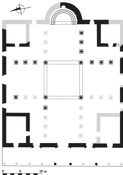
3. Церковь Пророков, апостолов и мучеников в Гересе (Джараш). План
