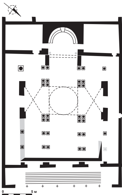
5. Храм свв. Сильвана и Фортунага в Суфетуле. План
