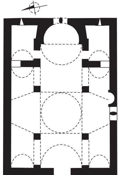
8. Храм в Ибрале (Йешилдере). План
