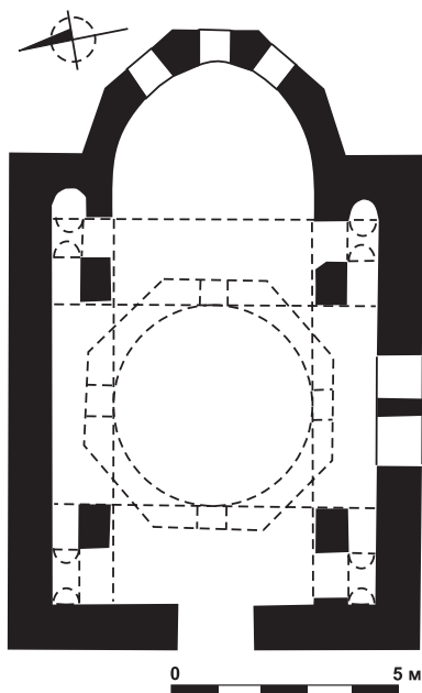
10. Храм в Антигусе (Йешилчурте). План
